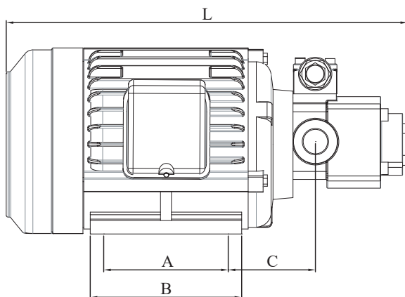
RBB-22 直插式電機組尺寸圖表 (CONNECT DIRECTLY)
